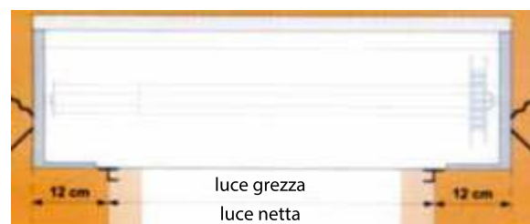
CASSONETTO STANDARD SEZIONE FRONTALE
